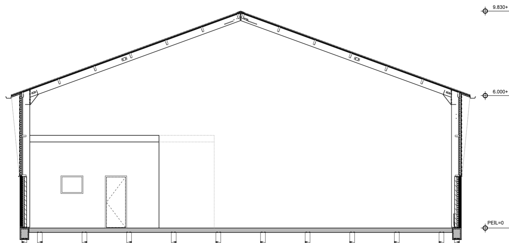
DOORSNEDE
